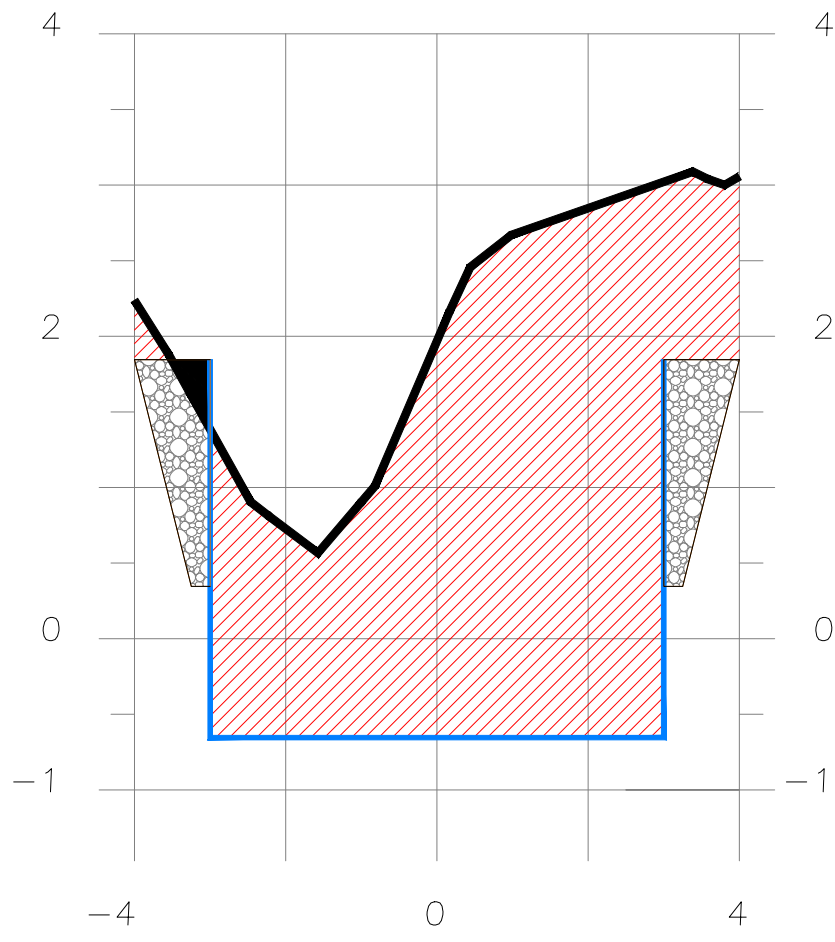
SECCION 3+285
