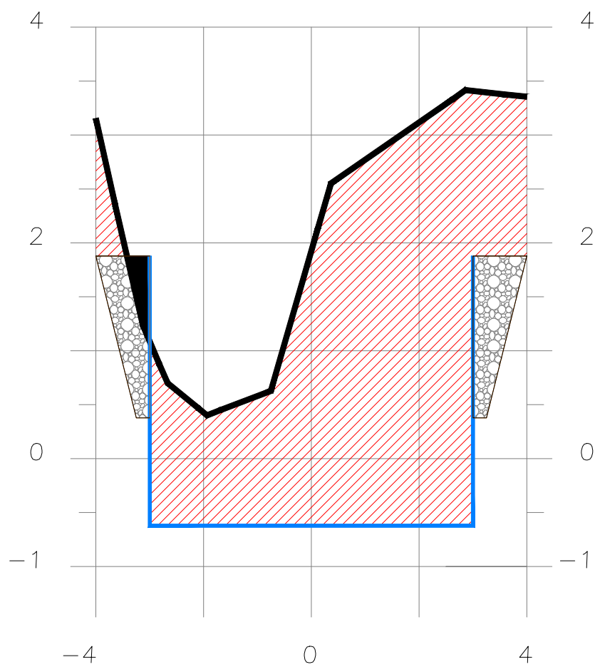
SECCION 3+210
