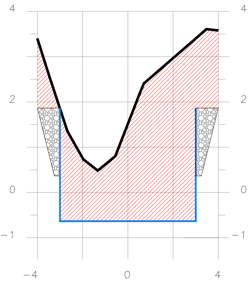
SECCION 3+240
