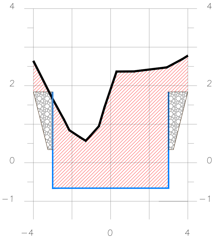
SECCION 3+300
