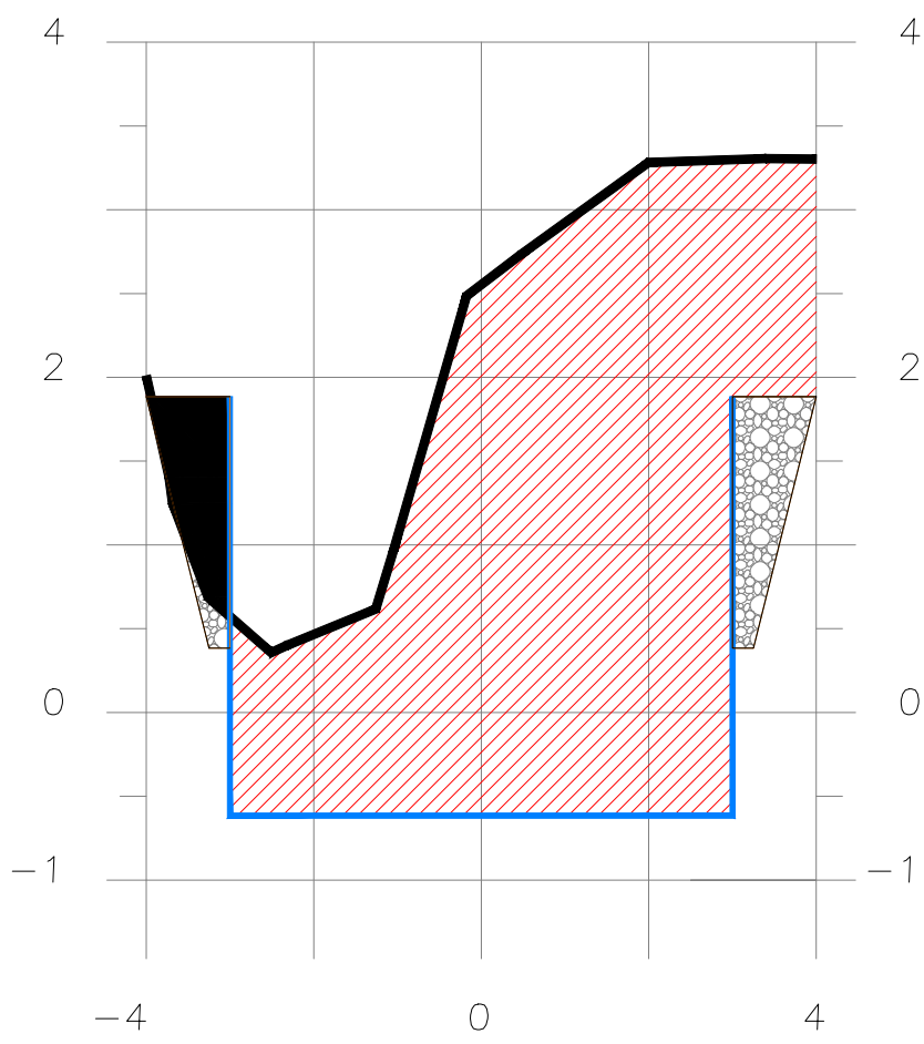
SECCION 3+195
