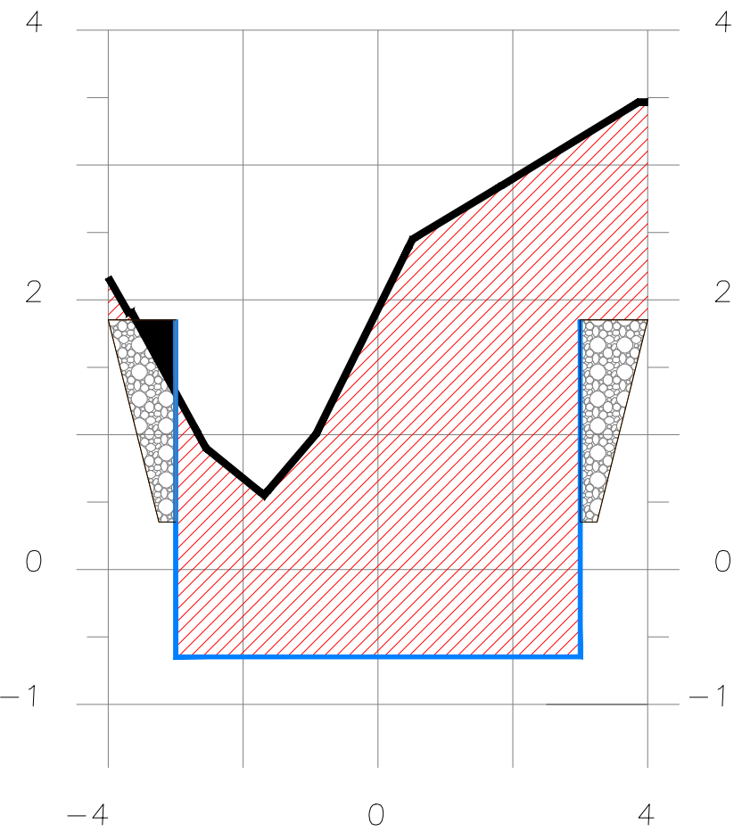
SECCION 3+270
