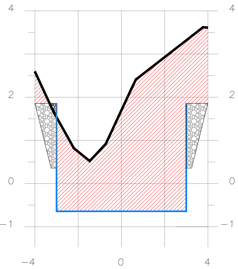
SECCION 3+255
