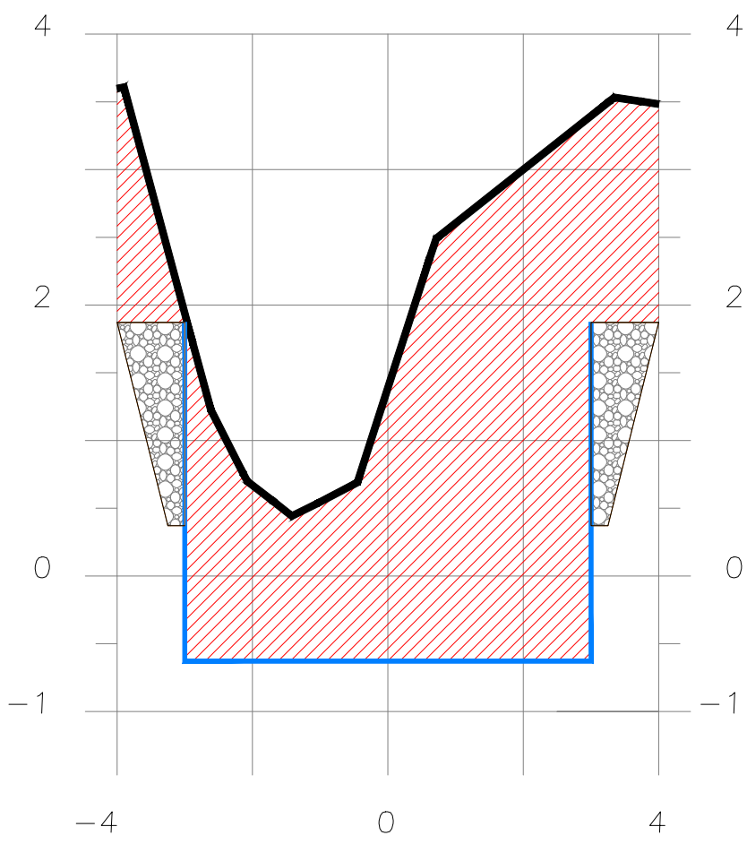
SECCION 3+225
