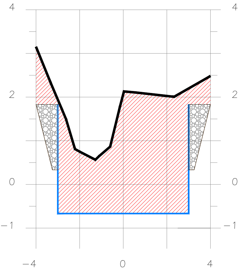
SECCION 3+315
